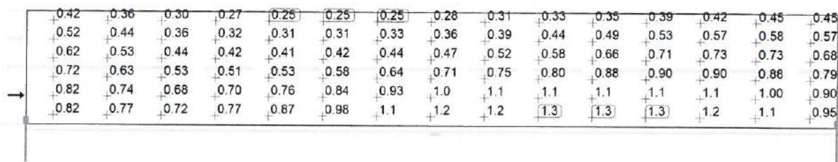
Observator 1: Valoarea de întreținere, densitatea luminii cu carosabil uscat [ \text{cd}/\text{m}^2 ] (Raster valoric)
