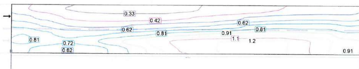
Observator 2: Valoarea de întreținere, densitatea luminii cu carosabil uscat [ \text{cd}/\text{m}^2 ] (Linii Isolux)
